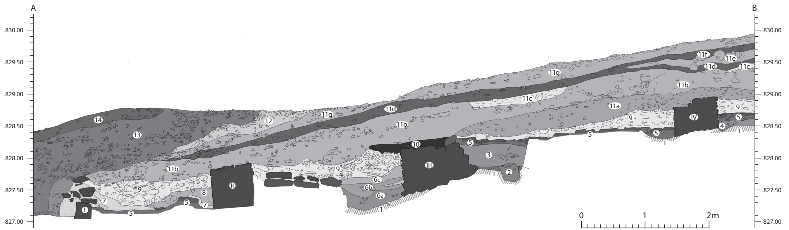
Abb. 4 Ältere Wohnbebauung westlich des Peristylhauses 2, Profilschnitt A/B 2008
