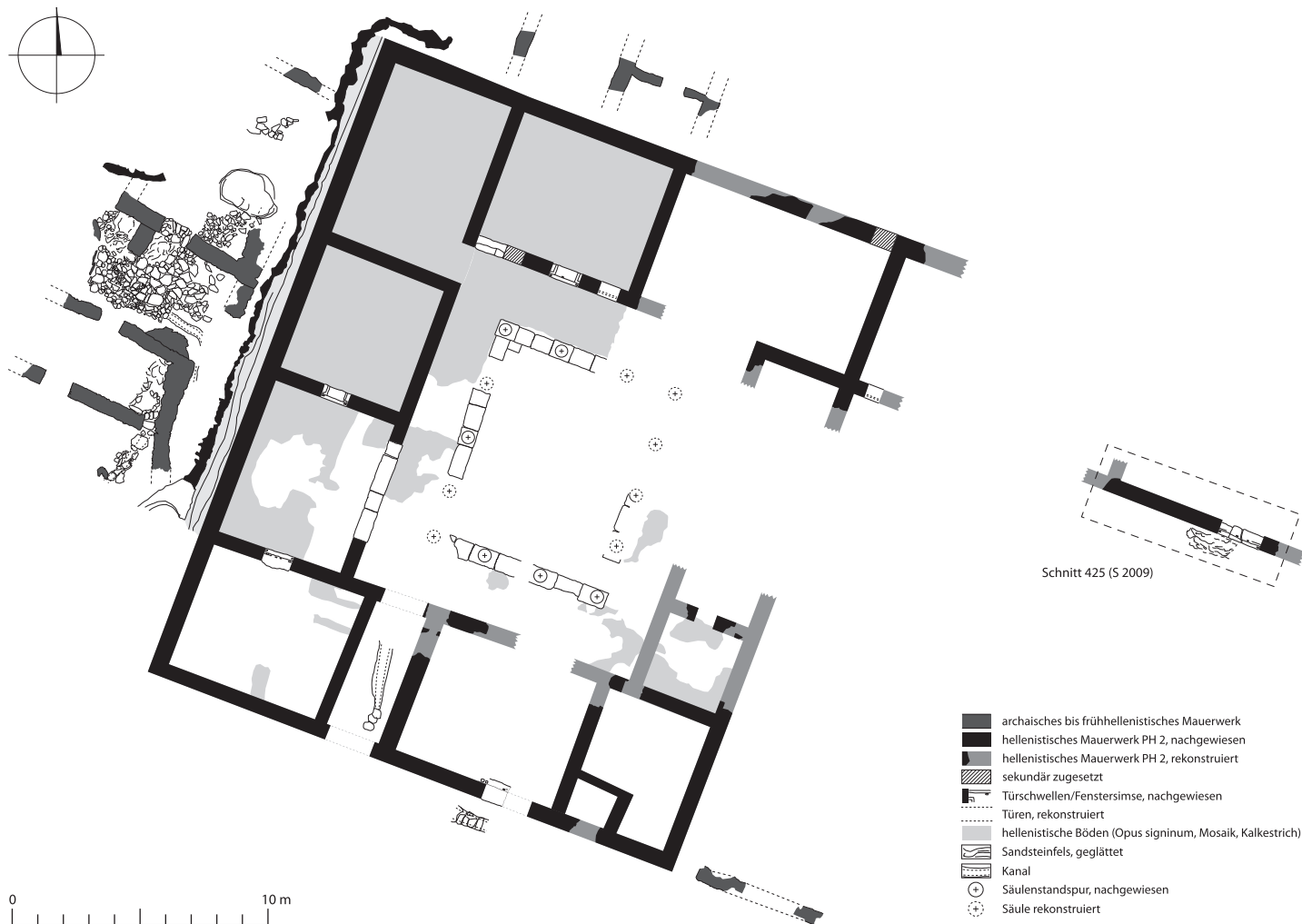
Abb. 2 Peristylhaus 2, antike Phasen, schematischer Plan 2009
