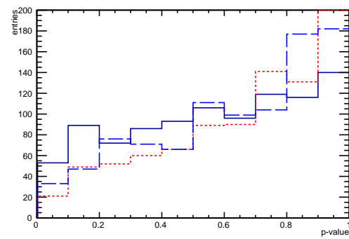
(d) 2nd order Chebychev polynomial
